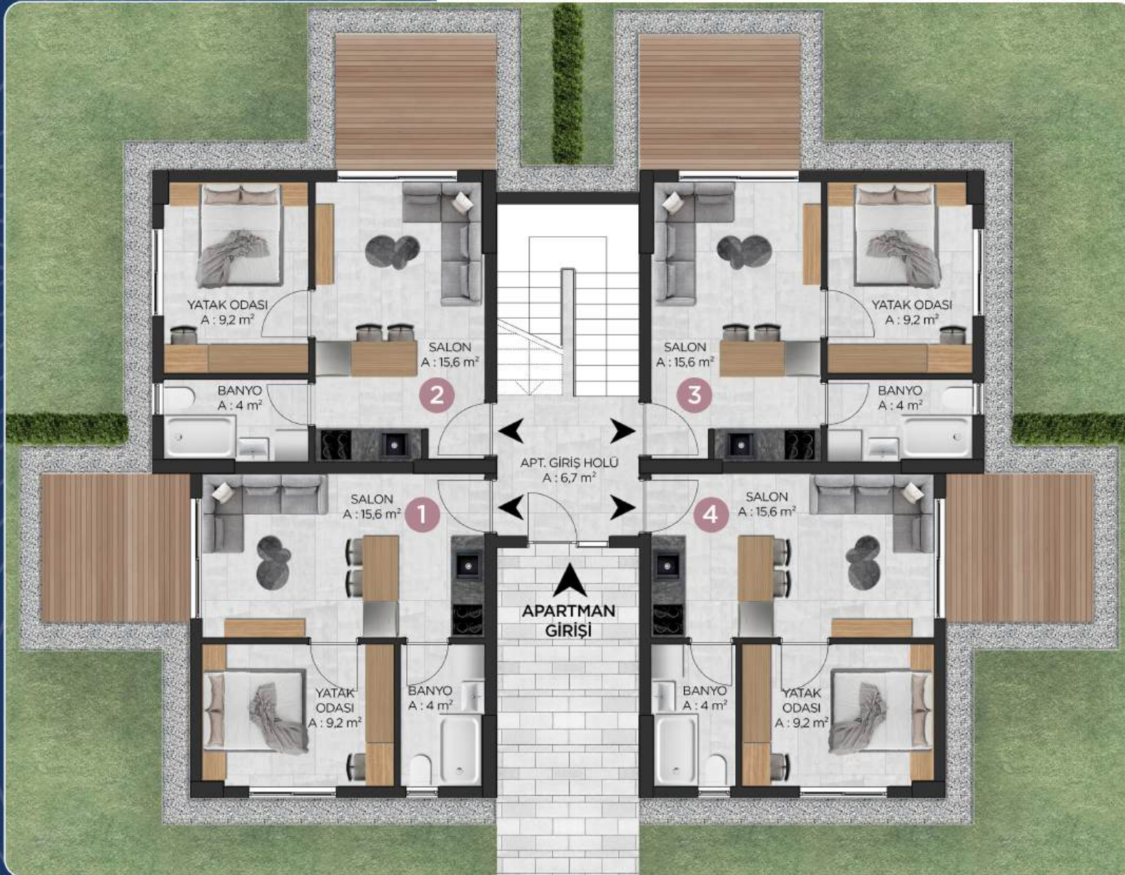
A-B BLOK ZEMİN KAT PLANI
