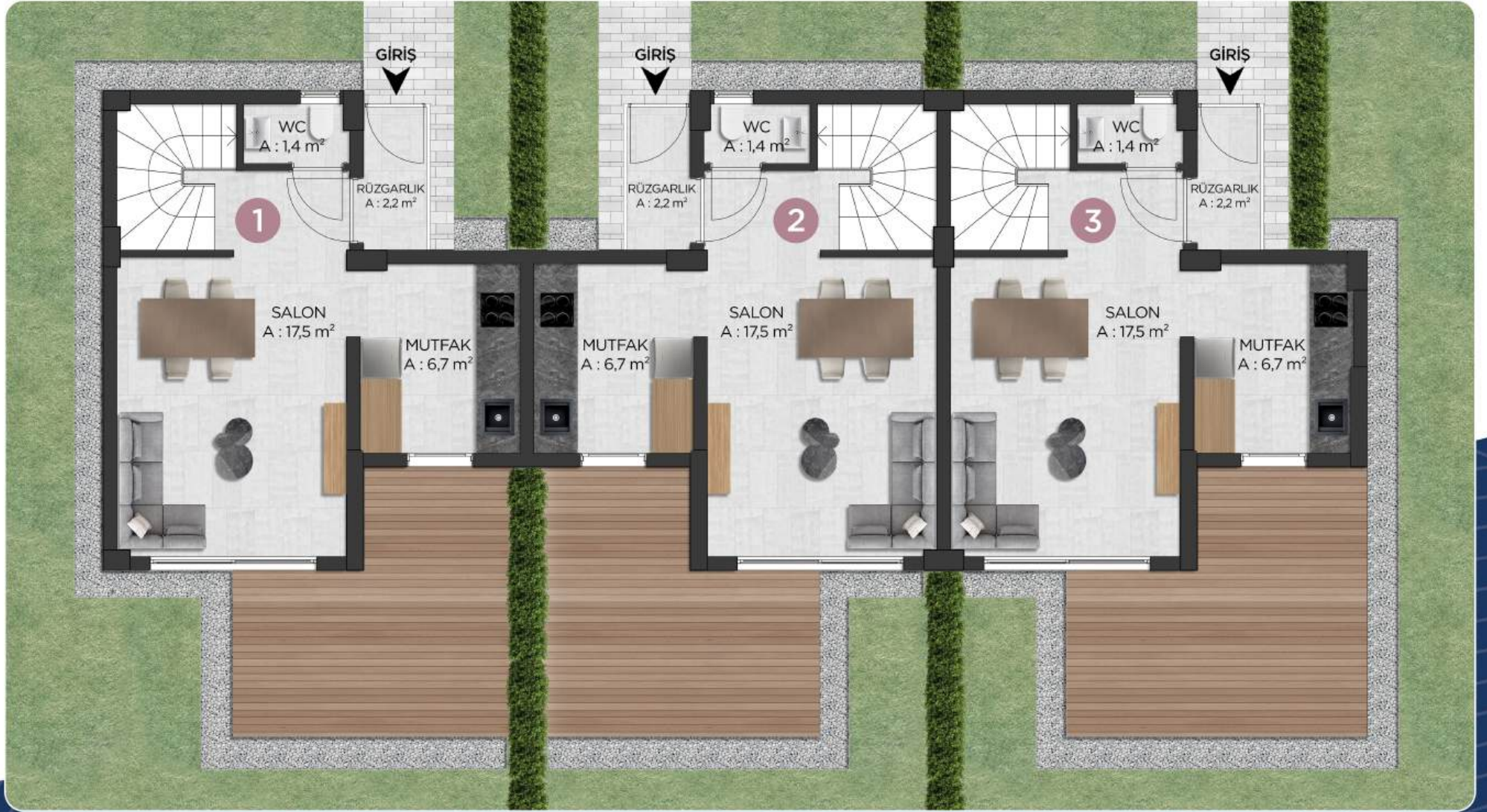
G BLOK ZEMİN KAT PLANI
