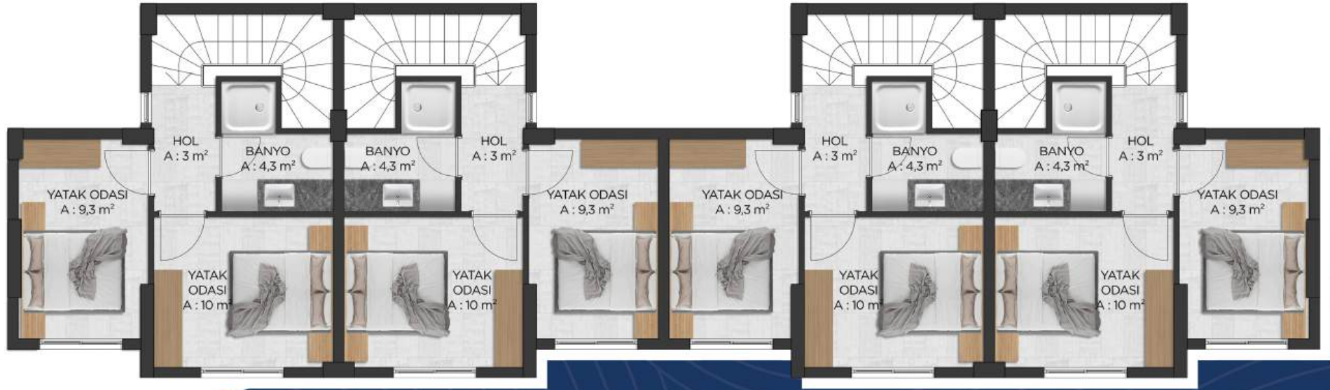
C-D-F BLOK 1. KAT PLANI
