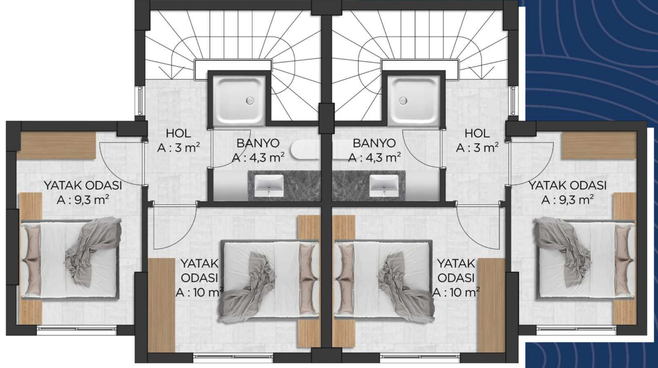
E BLOK 1. KAT PLANI
