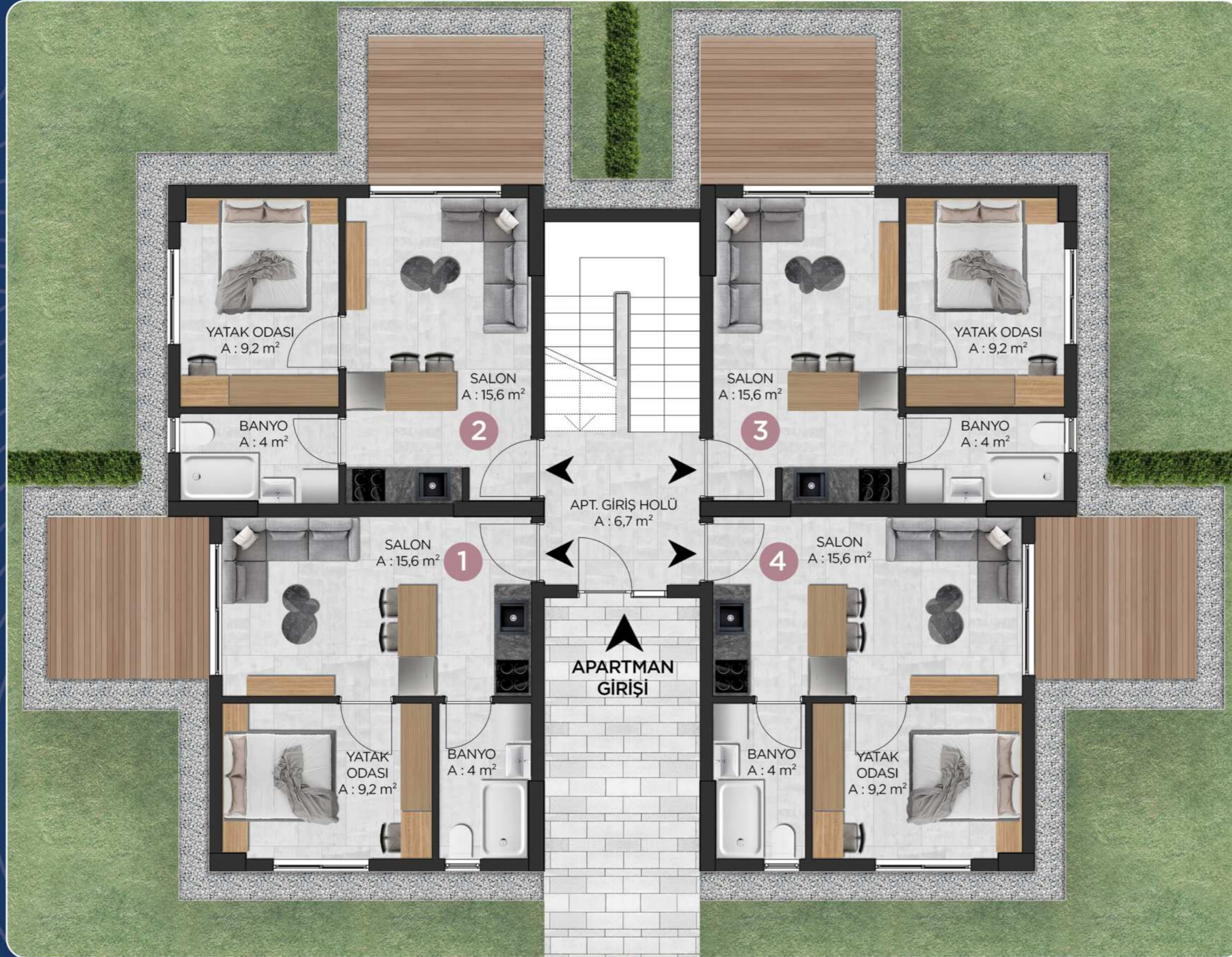
A-B BLOK ZEMİN KAT PLANI
